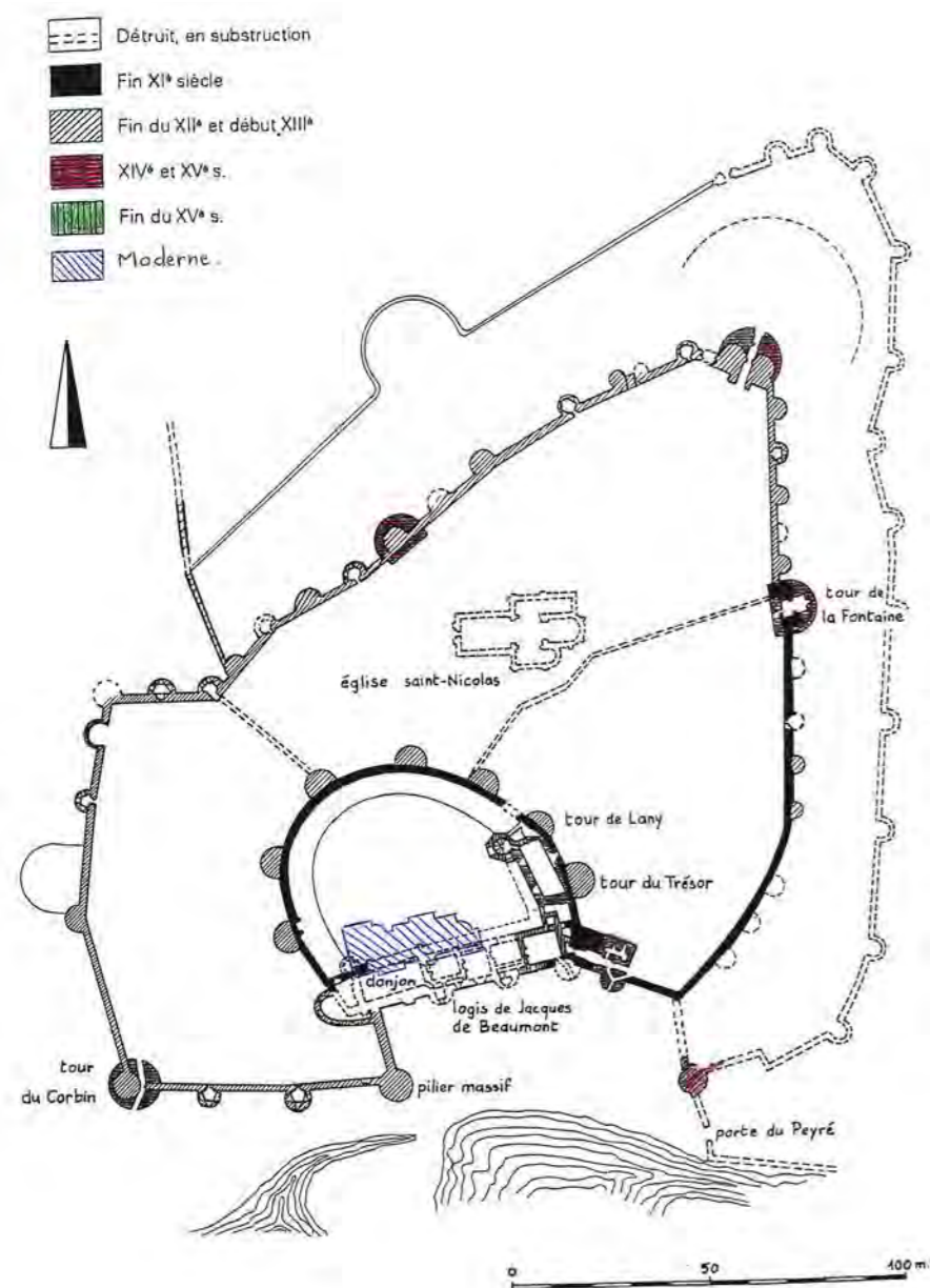
Plan du Château de Bressuire et datation des différentes parties de l'ensemble
