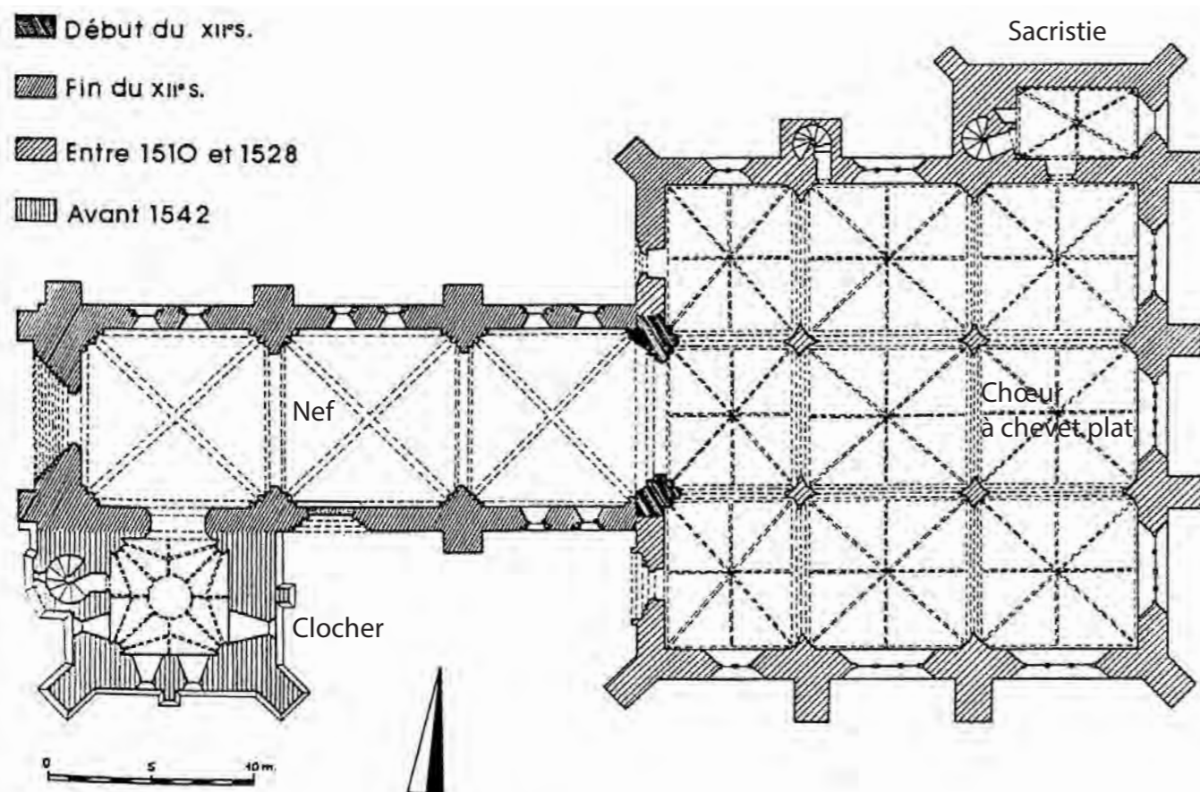
Plan de l'église Notre-Dame et datation des différentes parties de l'édifice Source : "Poitou gothique", Yves Blomme, Paris, 1993
